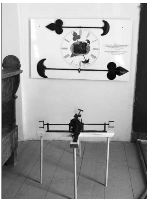
A nagyvárad-újvárosi templom órájának mánusai
